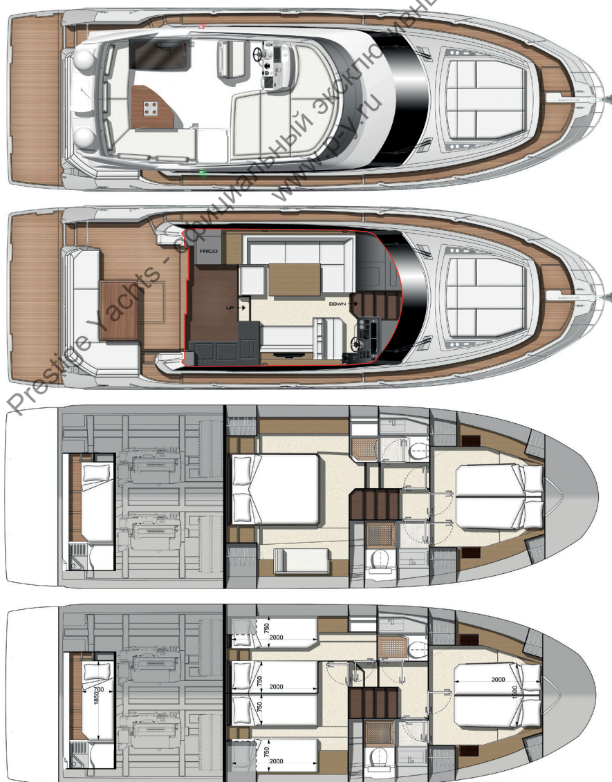
Версии с 2 и 3 каютами
